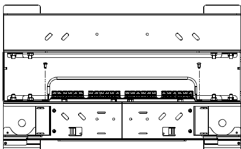
上面図
